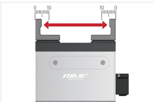
图 4 (单位 mm)
